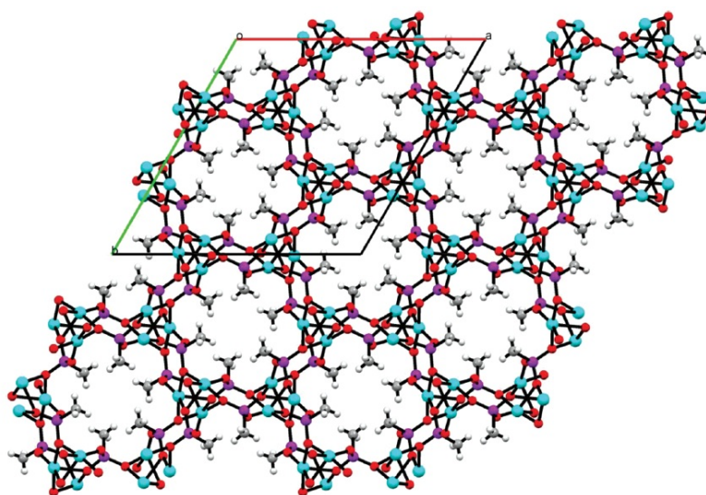
Рисунок 18. Структура \beta -Cu(O 3 PCN 3 ) с гидрофобными каналами, метильные группы повернуты в центр каналов (C=серый, O=красный, H=белый, P=фиолетовый).
