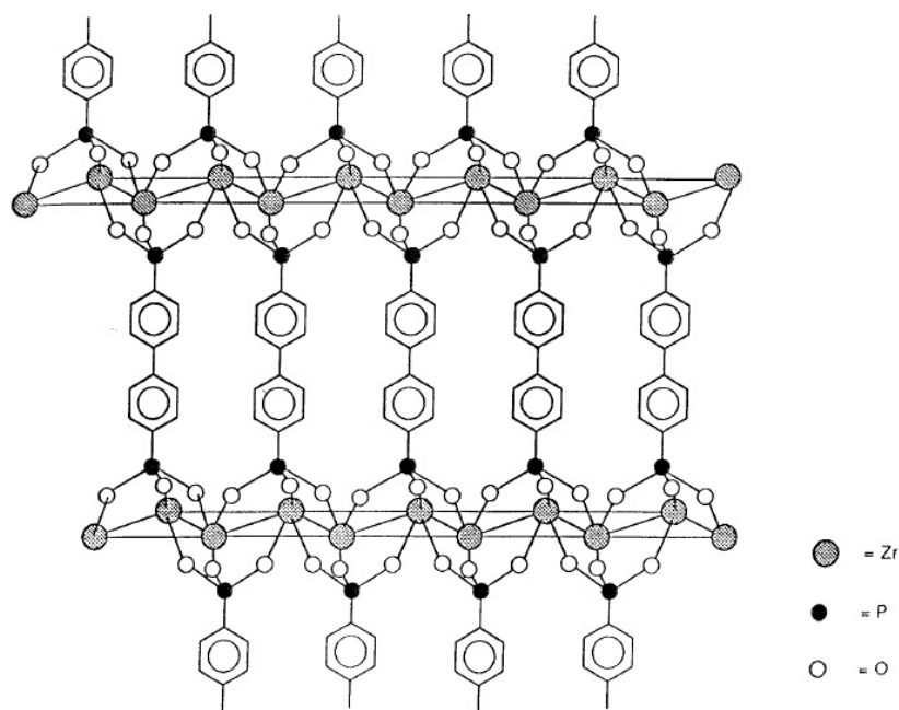
Рисунок 5. Схематическое представление структуры Zr(O_3PC_6H_4C_6H_4PO_3) , показывающее поперечную сшивку слоев, при которой не может быть образована микропористость.
