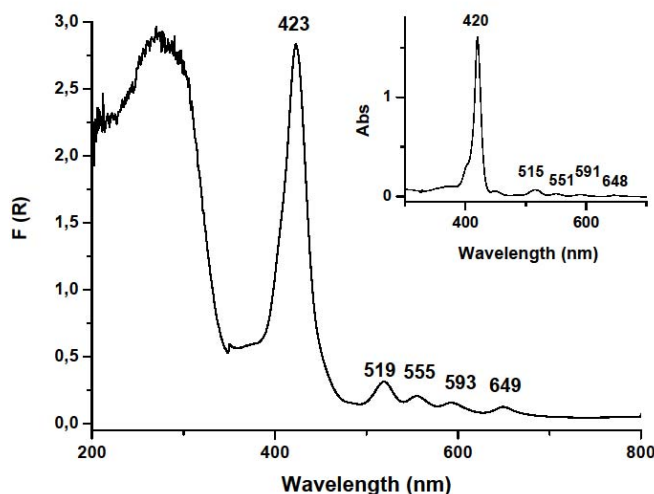
Рисунок 113. Спектр диффузного отражения гибридного материала 2H-12d@70TiO 2 . На вкладке справа электронный спектр поглощения в хлороформе свободного порфирина 2H-11d .
